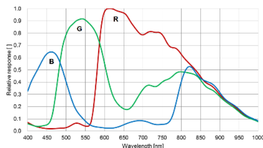
MV-CH089-10UC 量子效率
