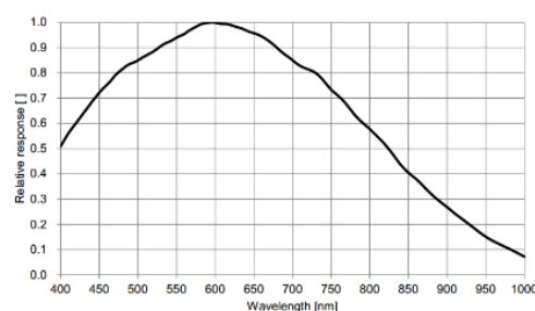
MV-CH089-10UM 量子效率
