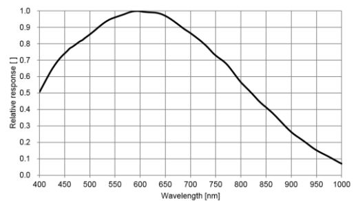
MV-CS050-10GM-PRO 量子效率
