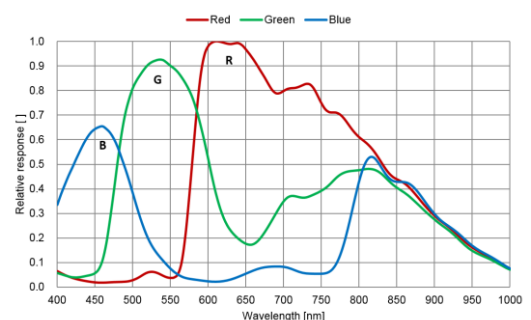
MV-CS050-10GC-PRO 量子效率
