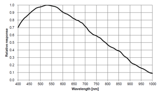
MV-CU060-10GM 响应曲线
