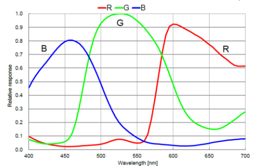
MV-CU060-10GC 响应曲线
