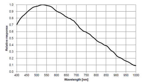
MV-CU060-10UM 量子效率
