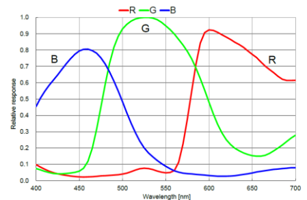
MV-CU060-10UC 量子效率
